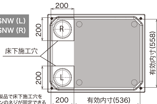
タテ引き排水トラップ [品番:YT-SNW]スノーホワイト
