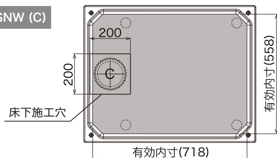
BS-8064SNW (L) BS-8064SNW (R)
