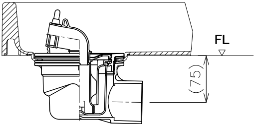
設置例:ヨコ引きトラップ 【有色】XT-SNW 【透明】XT-C-SNW
