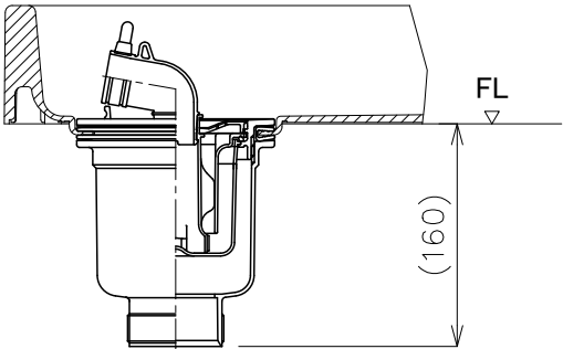
設置例:タテ引きトラップ 【有色】YT-SNW
