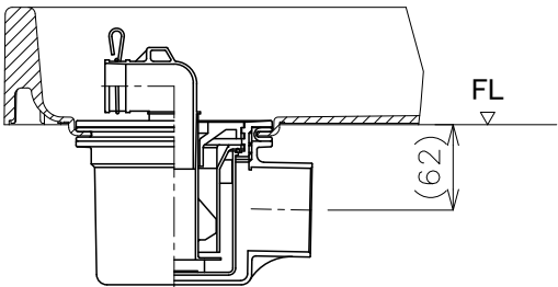
設置例:ヨコ引きトラップ 【透明】CT-SNW
