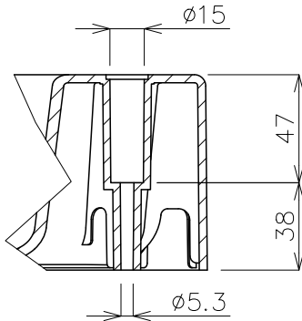
断面 C-C(S=1:3)
