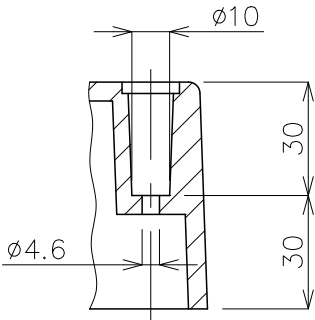
断面 B-B(S=1:2)
