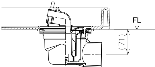
設置例:ヨコ引きトラップ 【有色】XT-SNW 【透明】XT-C-SNW
