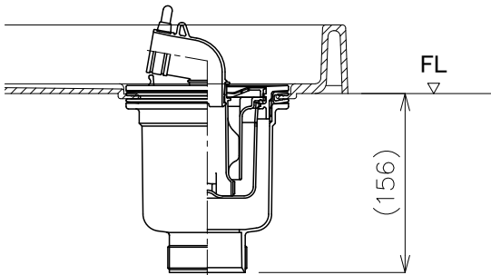
設置例:タテ引きトラップ 【有色】YT-SNW
