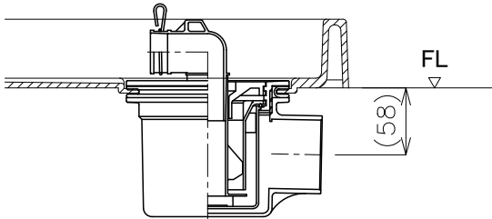
設置例:ヨコ引きトラップ 【透明】CT-SNW
